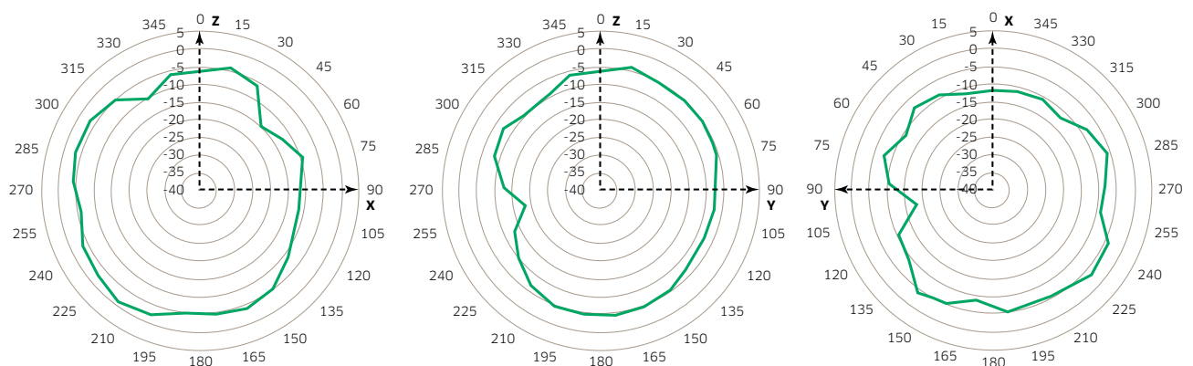
Figure 1. OmniAccess AP1201 BLE antenna pattern
